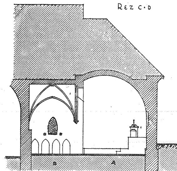
Obr. 26. Rez Prívinozho kostola v Nitre. A. Apsis. B. Loď. Terajší stav.
