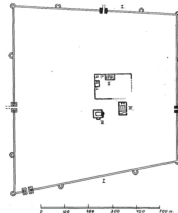
Obr. 187. Plán dvorce v Abobě u Šumna.
