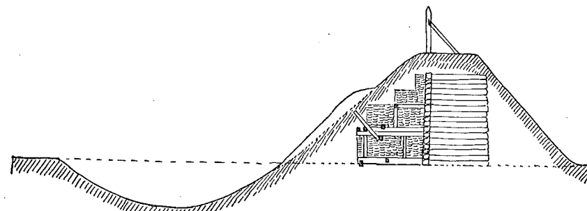
Obr. 184. Konstrukce valu v Bělgorodce.
