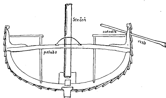
Obr. 125. Průřez vikinské lodi (podle W. Vogla).
