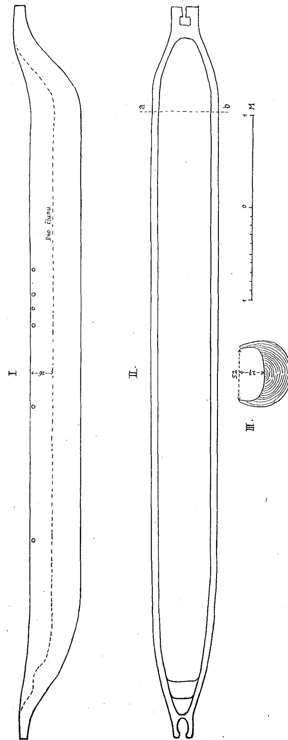
Obr. 122. Dřevěný člun vydlabaný z dubového kmene, nalezený v Labi u Kolína.
