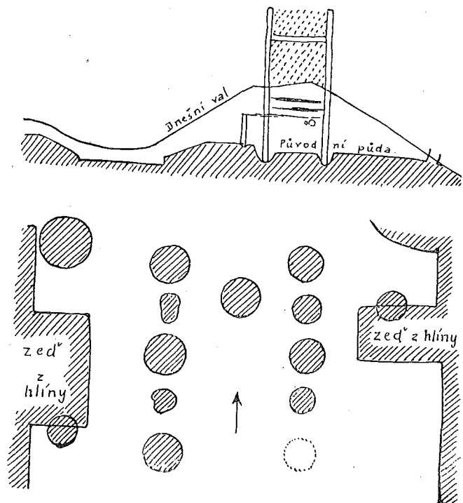
Obr. 183. Konstrukce valu a půdorys brány hradiště u Postupimě (K. Schuchardt).
