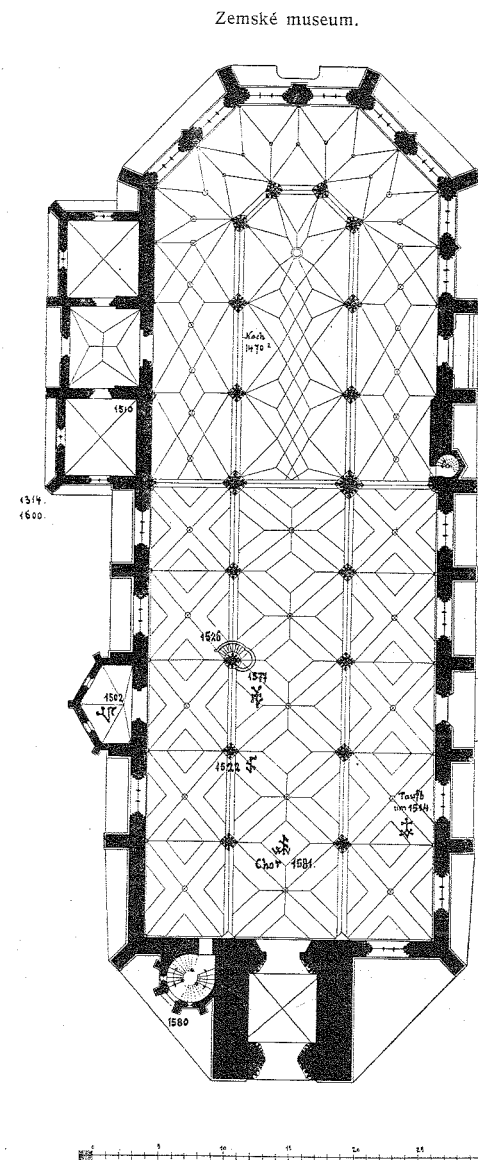
Obr. 20. Půdorys chrámu sv. Jakuba.
