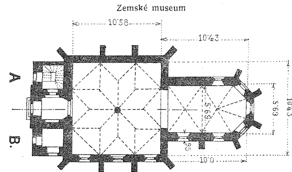
Obr. 4. Půdorys kostela sv. Mikuláše.
