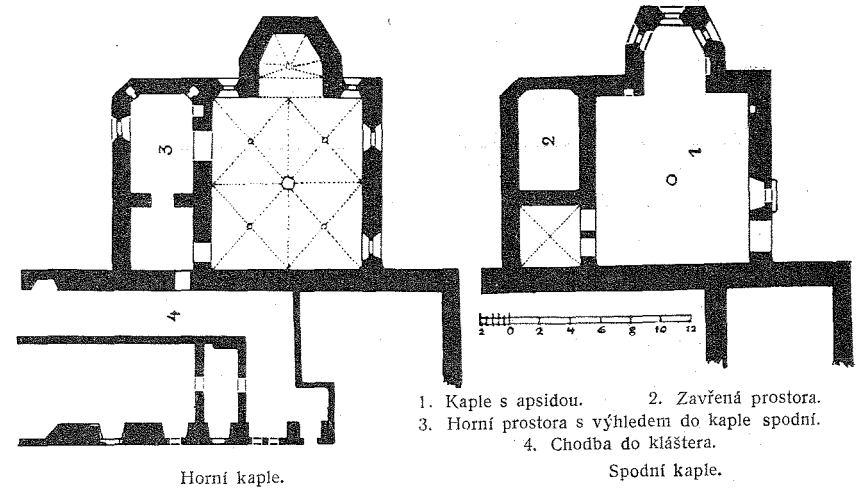
Obr. 5. Pádorys kaple P. Marie na Rybném trhu.
