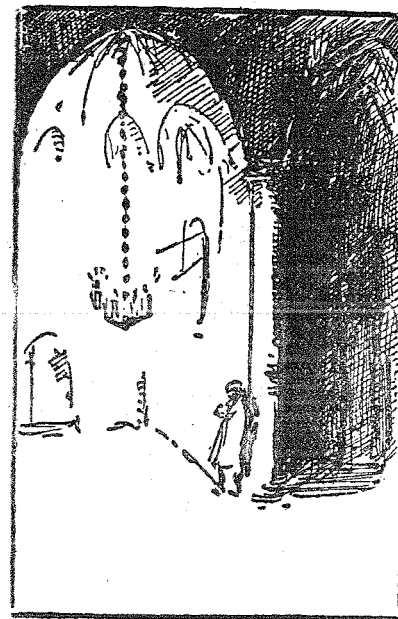
Galileo.
