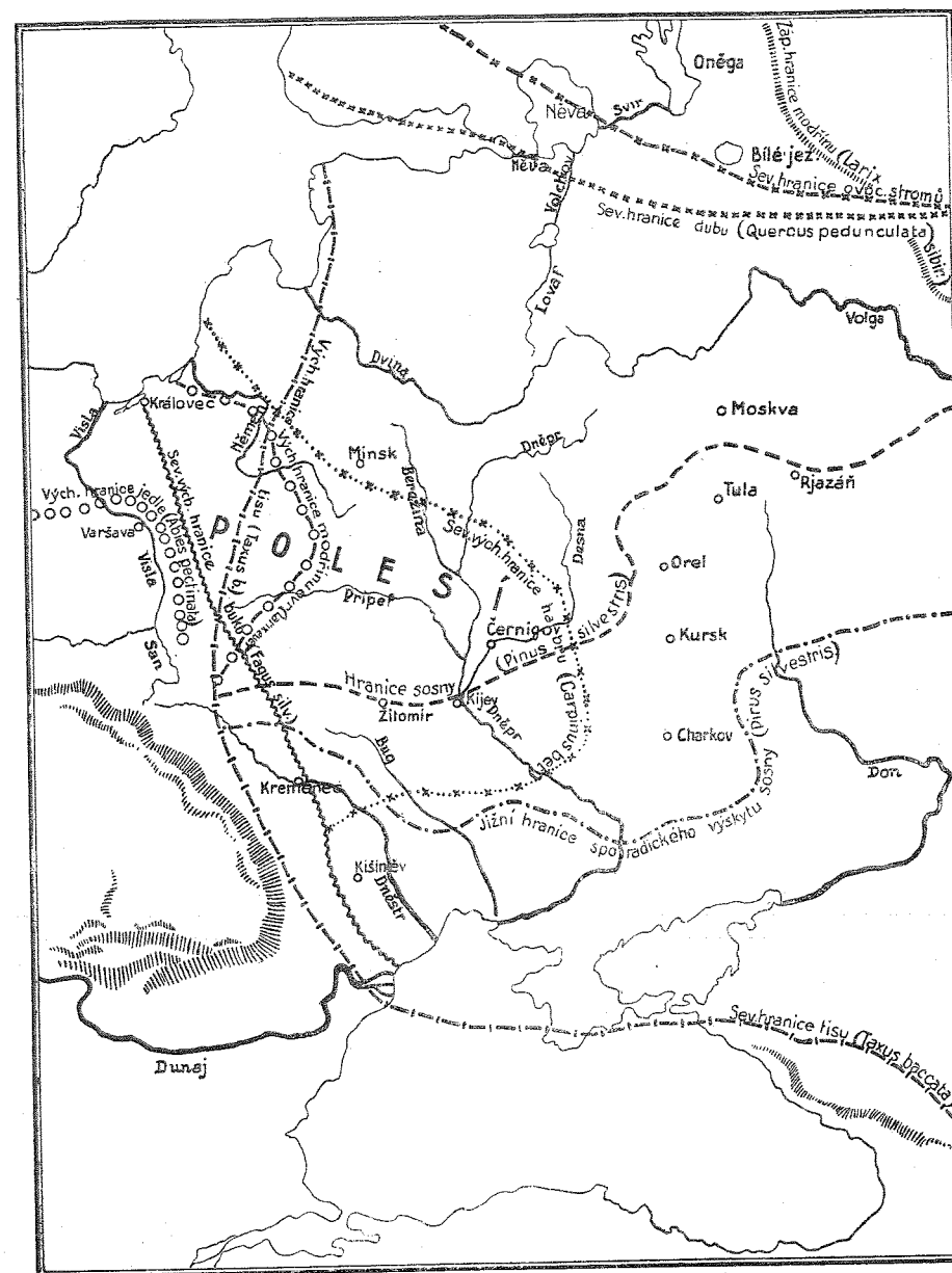
Rozšíření štmové vegetace v Rusku (podle Kuzněcova).
